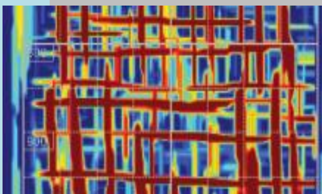
scan van wapening in betonplaat
